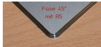
Fase 45° mit R5
